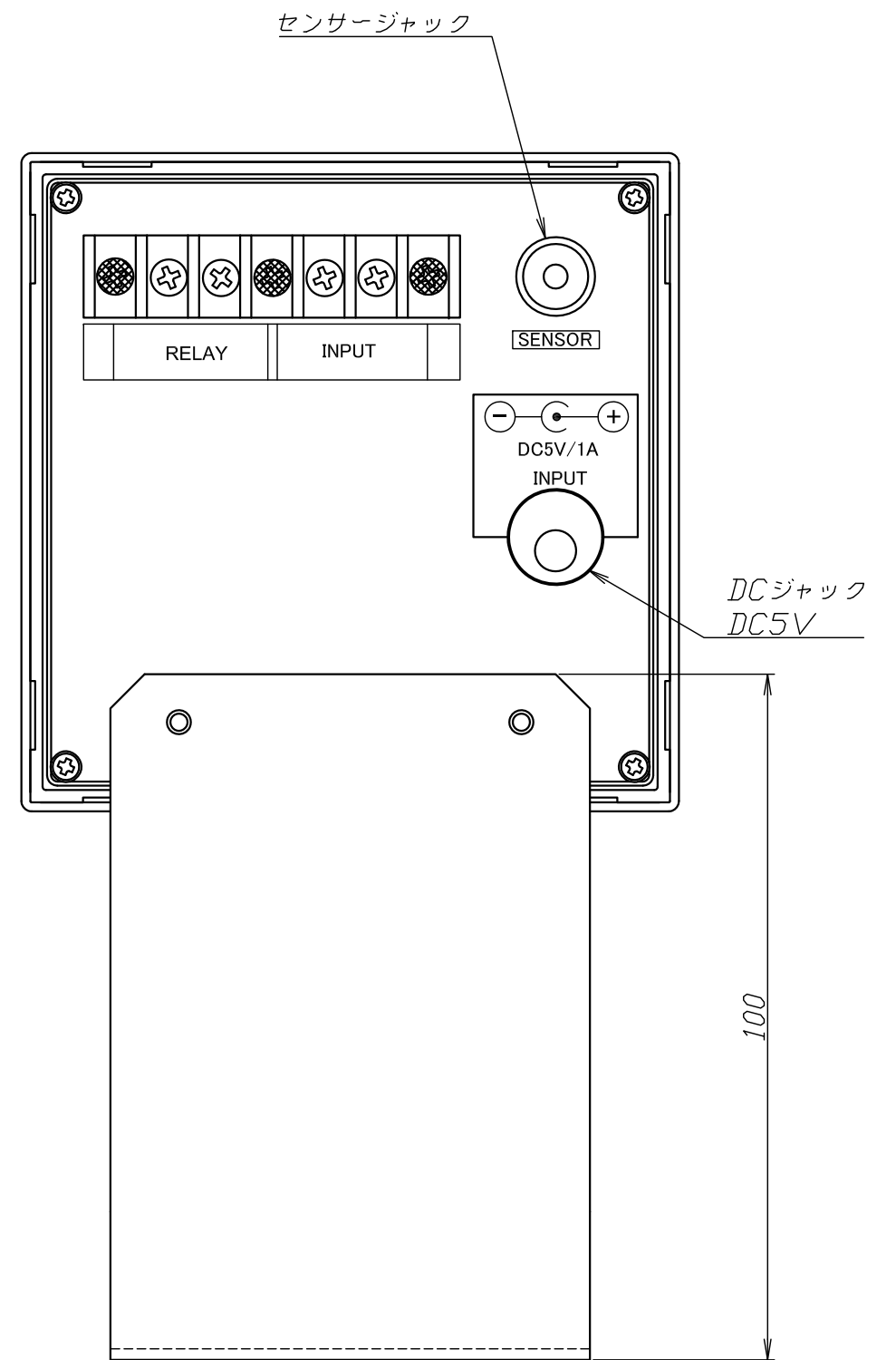
後面図
