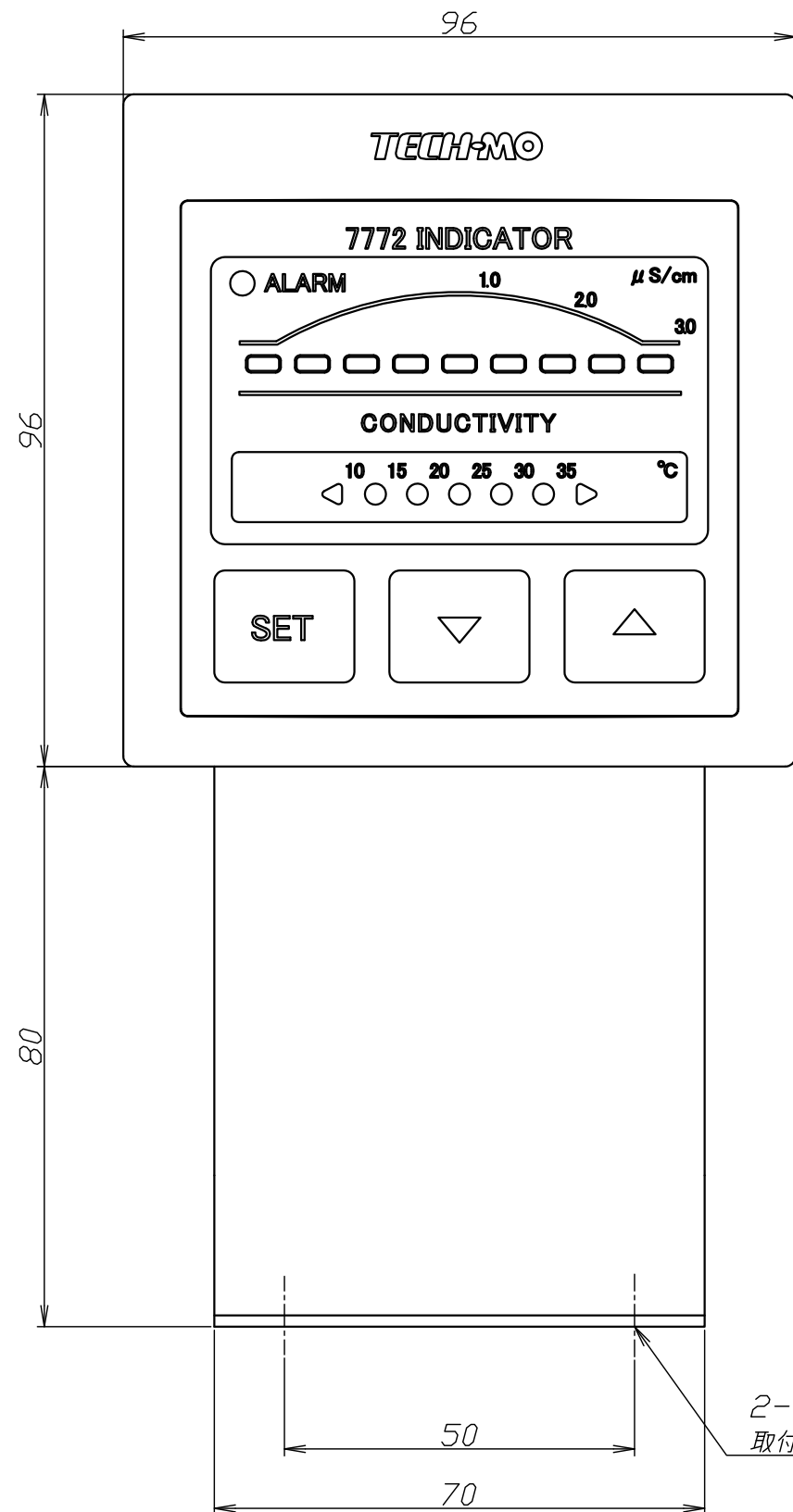
前面図
