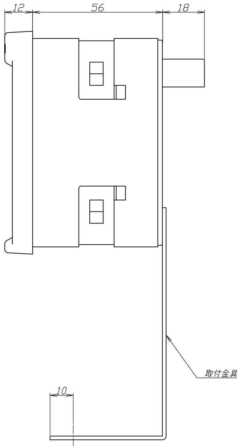
側面図
