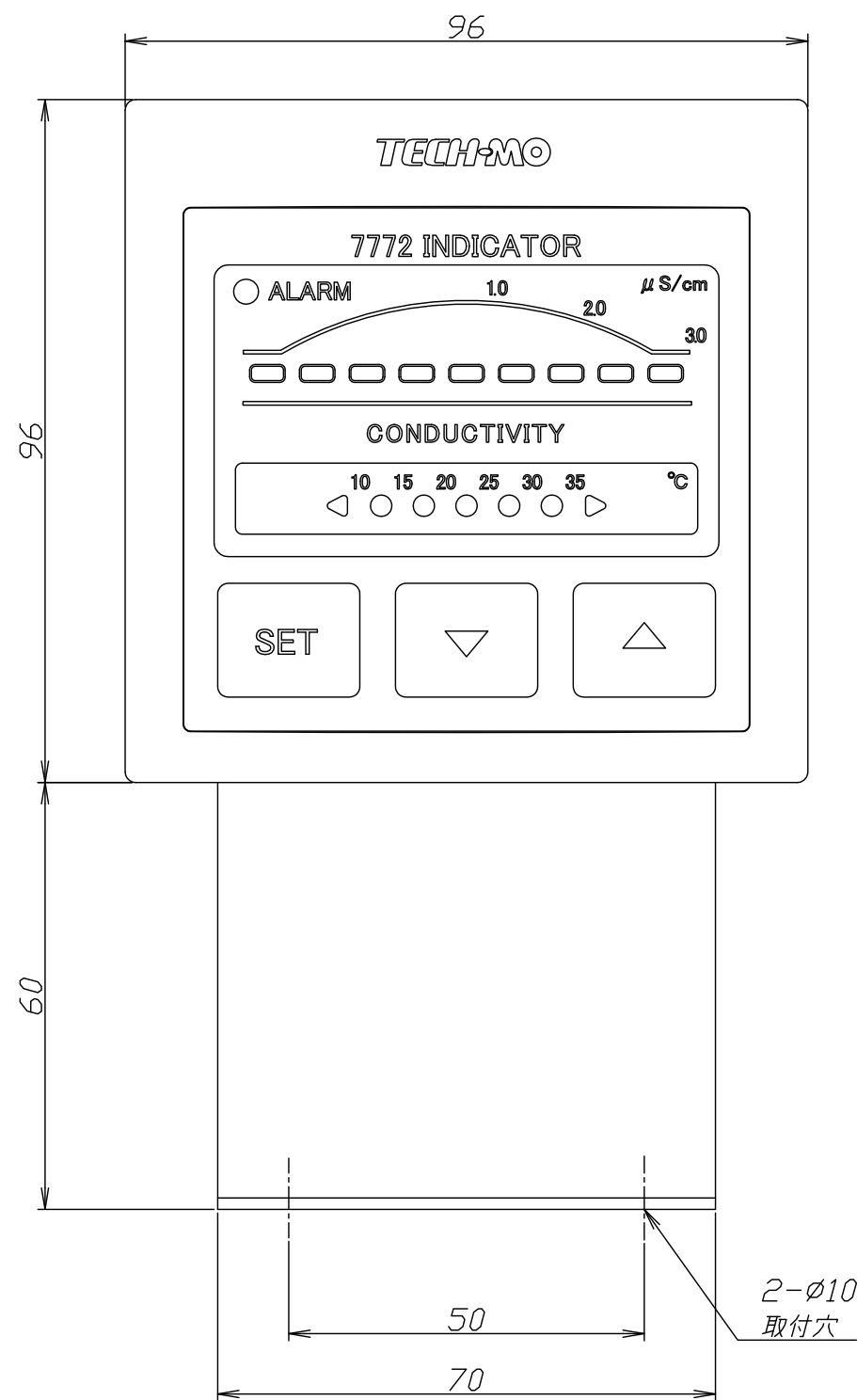
前面図
