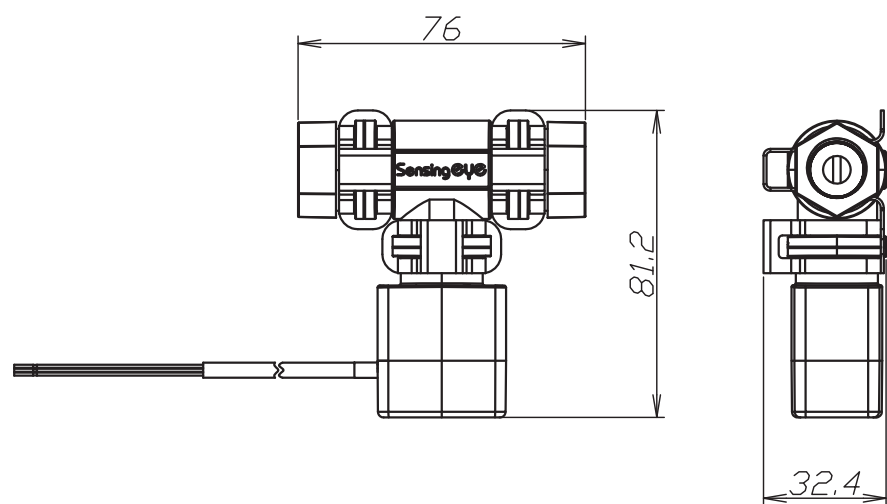
チーズ型接続 外形図
