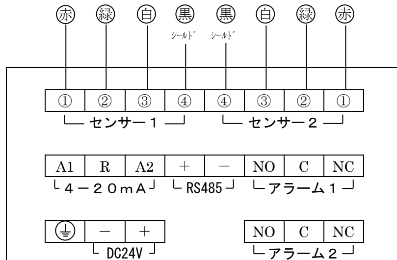
《7722-A202N 後面パネル視》
