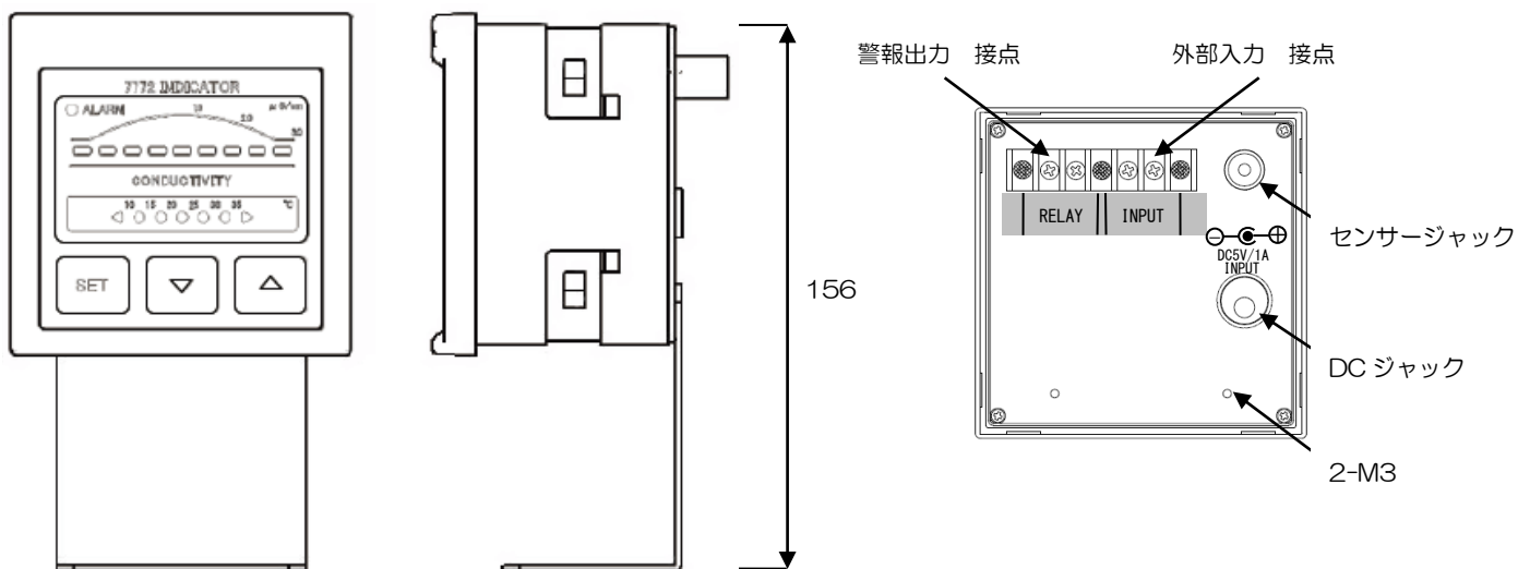
取付金具付き本体外形図
